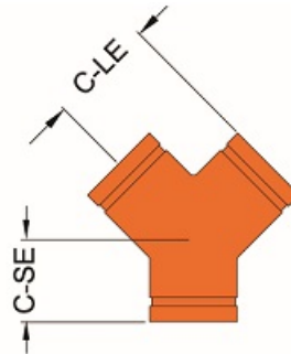
7137 True-Y
