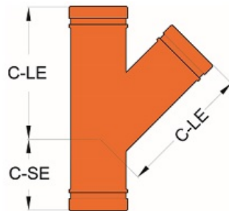
7130 45° Lateral
